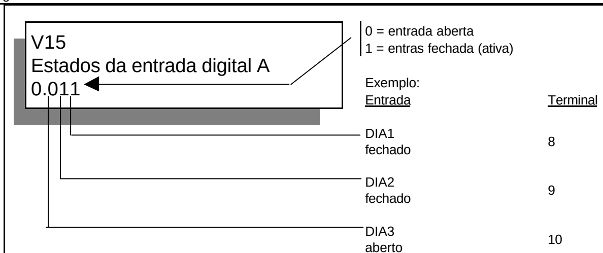
Figura 7-4 - Entradas digitais, Status grupo A
