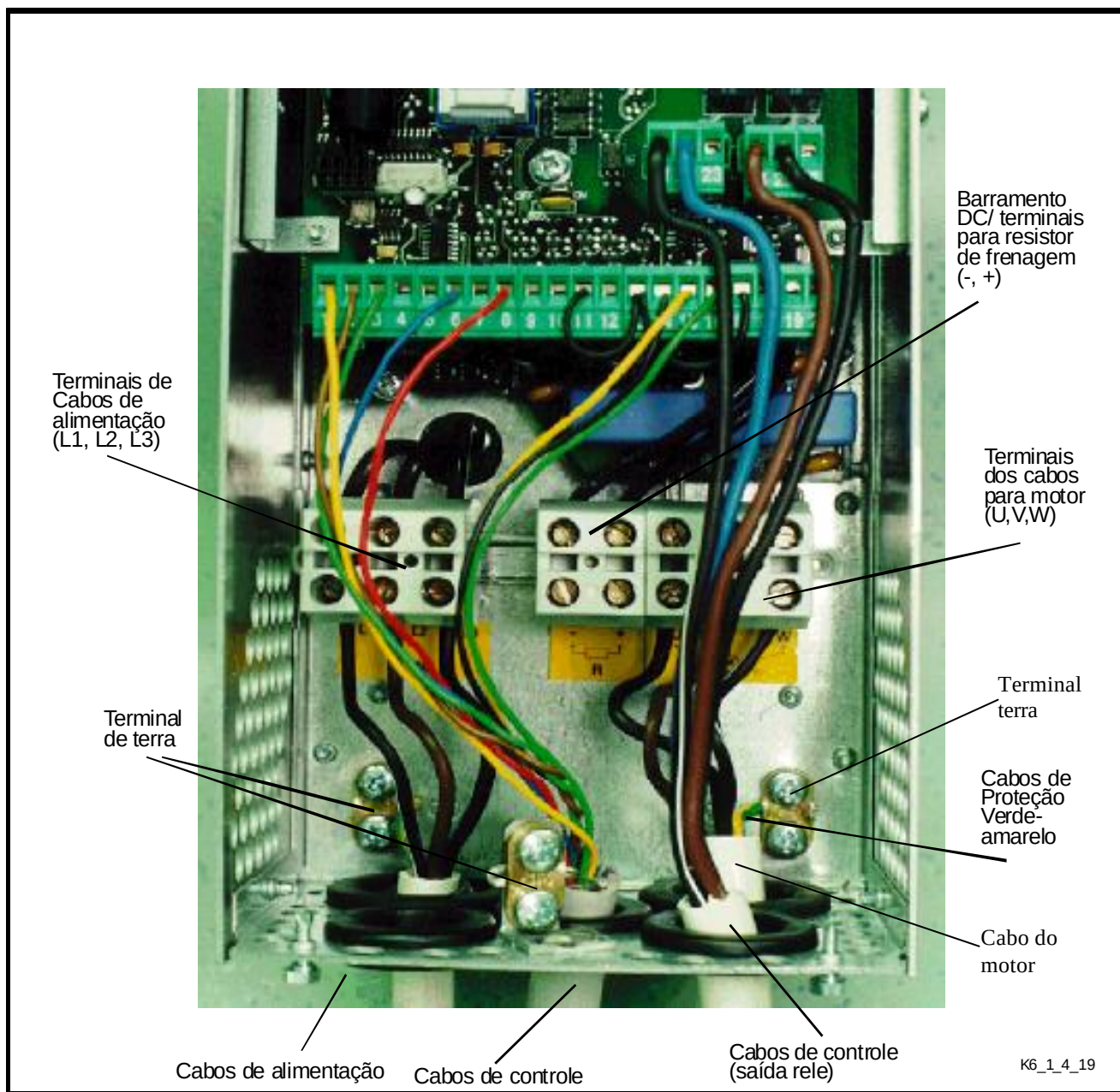
Figura 6.1.4-19 - Ligação para cabos do Vacon 4 - 11 CXS5 (EMC nível N)
