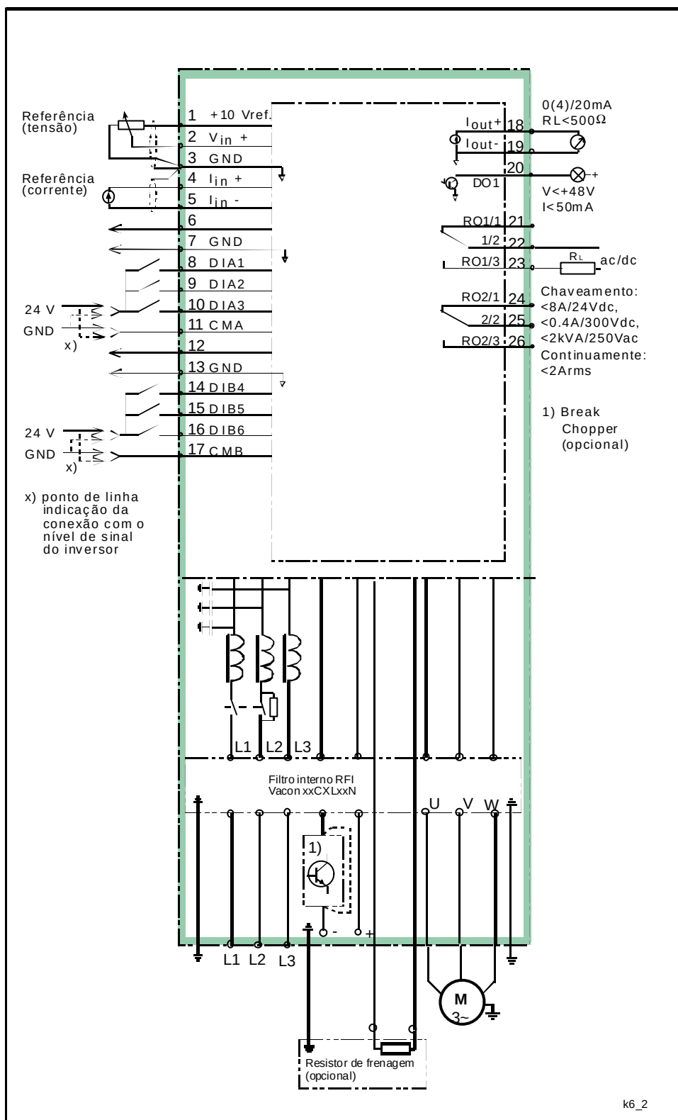
Figura 6-2 - Diagrama de conexões, linha CX (para unidade \geq M7 ) e série CXL (para unidades \geq M8 )
