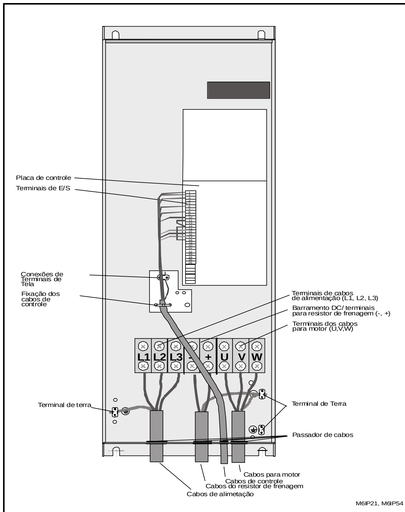
Figura 6.1.4-8 - Ligação para cabos do Vacon 18.5 - 45CXL4/CXL5 e 11 - 22 CXL2 (EMC nível N)
