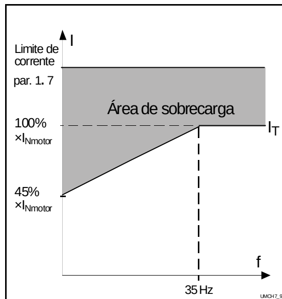
Figura 10.5.1-1 - Curva da Corrente térmica I_T do motor
