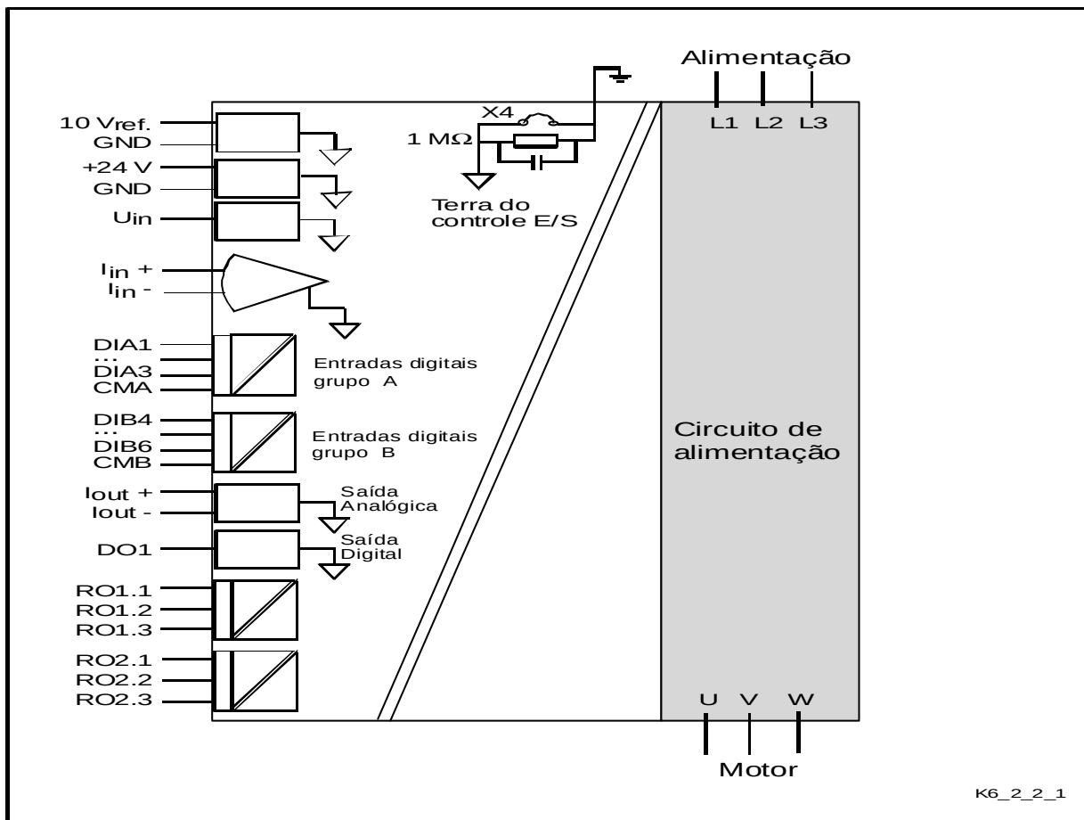
Figura 6.2.2-1 - Barramento Isolado
