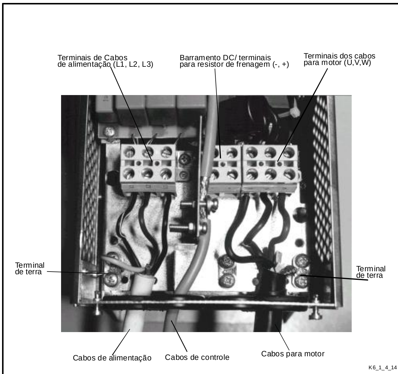
Figura 6.1.4-14 - Ligação para cabos do Vacon 2.2 - 45 CXL4/CXL5 (EMC nível I)
