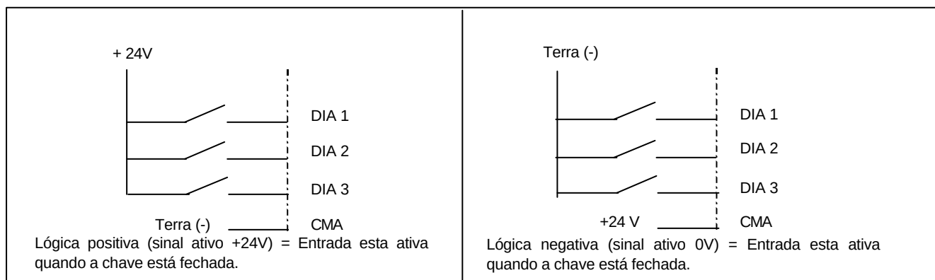
Figura 6.2.3-1- Lógica positiva / negativa
