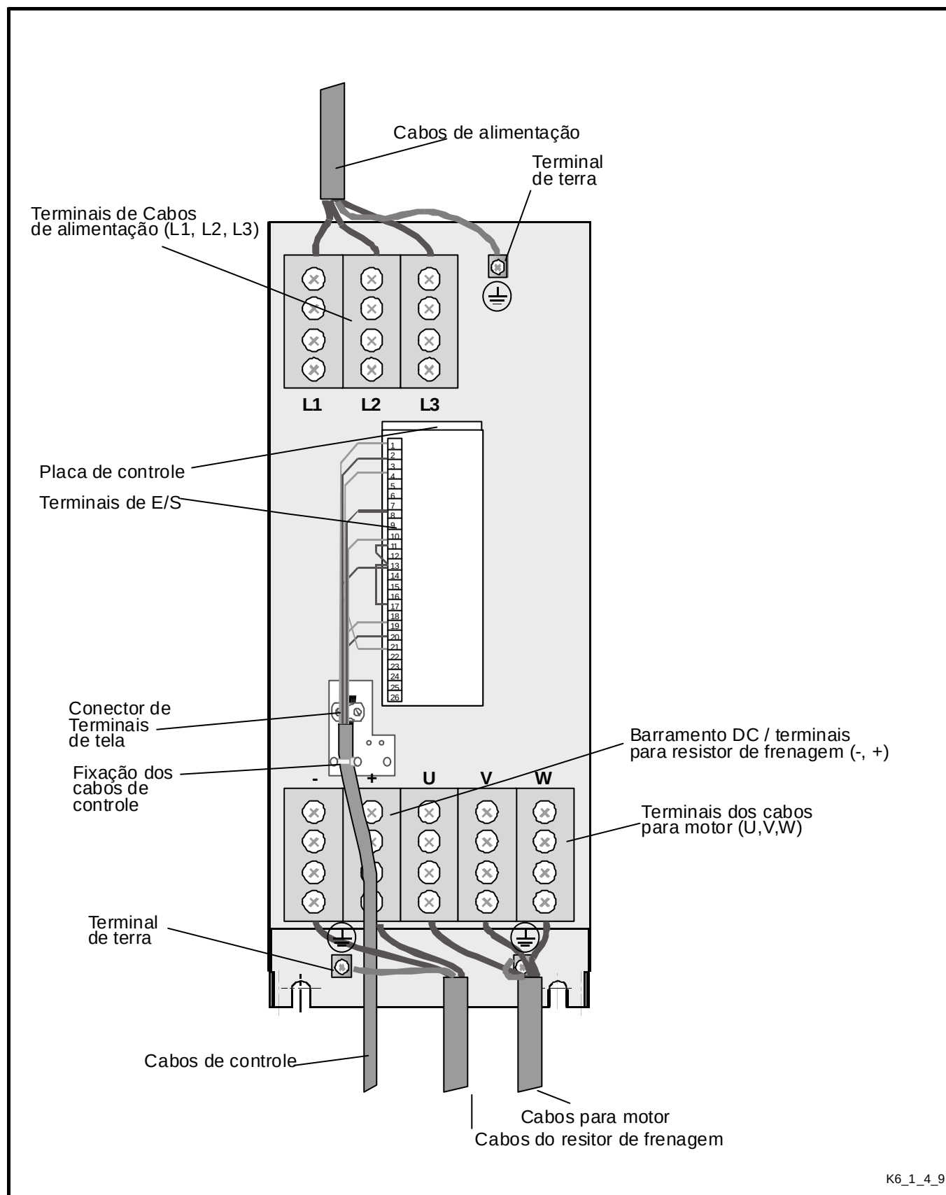
Figura 6.1.4-9 - Ligação para cabos do Vacon 55 - 90 CX4/CX5, 30 - 45 CX2 (EMC nível N)
