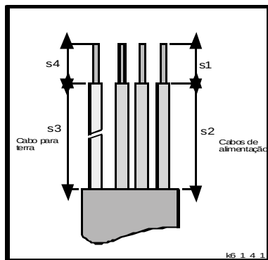
Figura 6.1.4-1 - Cabeamento do motor e da alimentação
