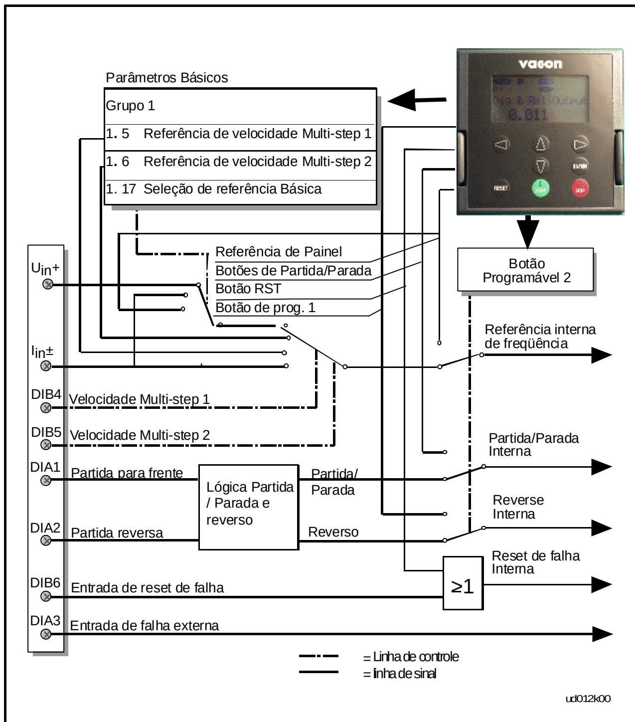
Figura 10.3 - 1 mostra a lógica de controle dos sinais de E/S e botões de navegação.
