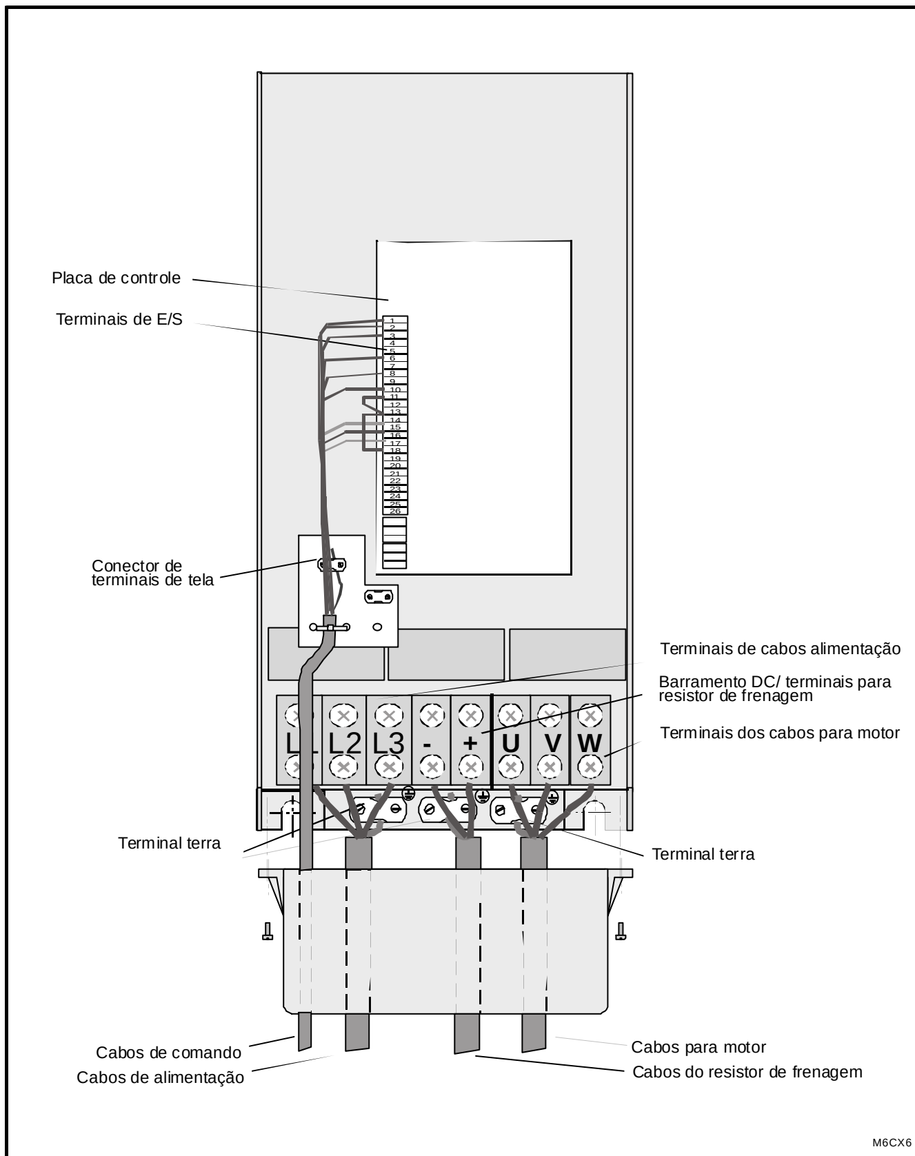
Figura 6.1.4-13 - Ligação para cabos do Vacon 30 - 75 CX6 (EMC nível N)
