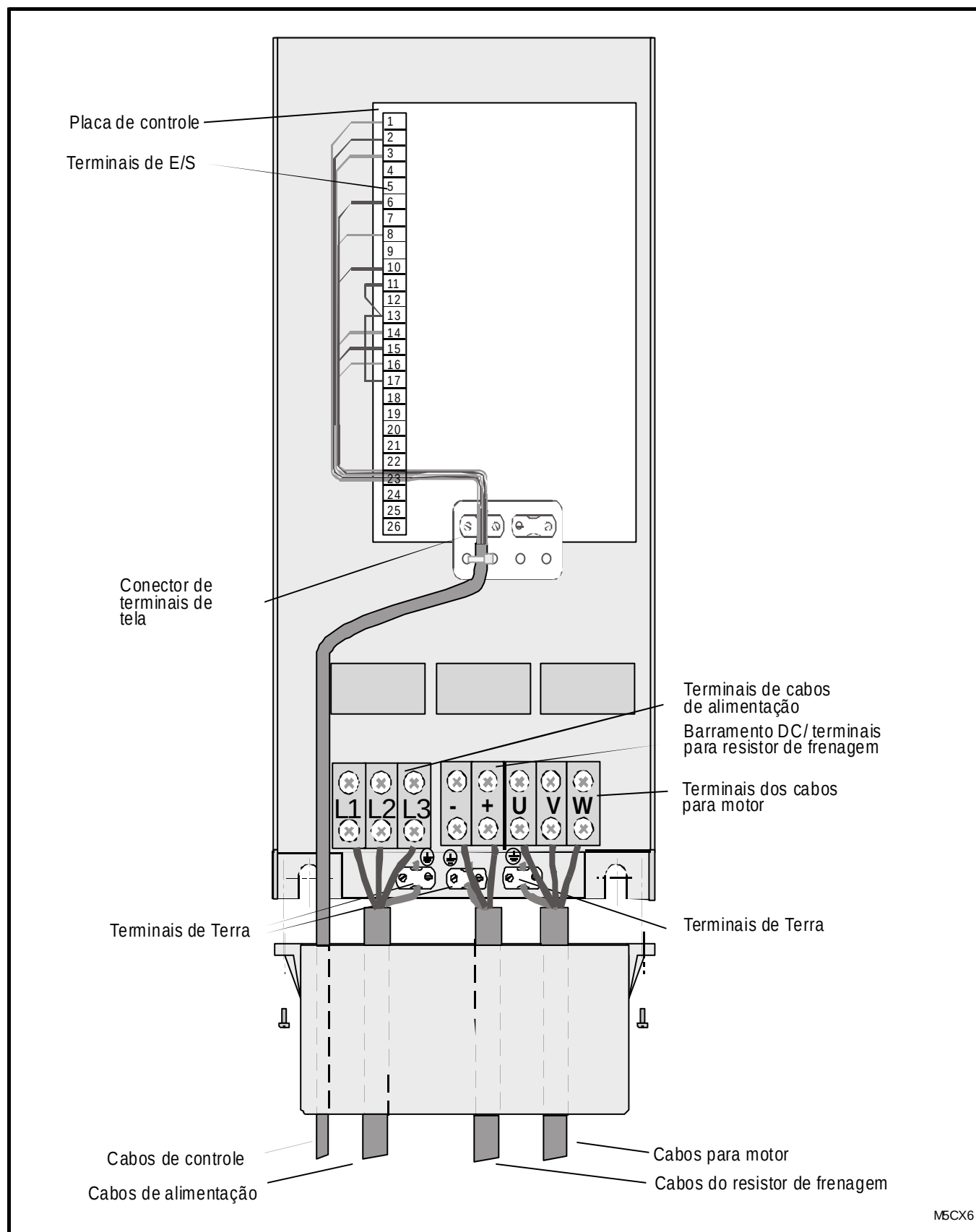
Figura 6.1.4-12 - Ligação para cabos do Vacon 2.2 - 22 CX6 (EMC nível N)
